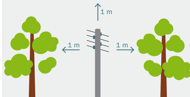
Abstände im Niederspannungsbereich
